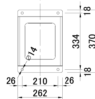
モニター固定用金具
